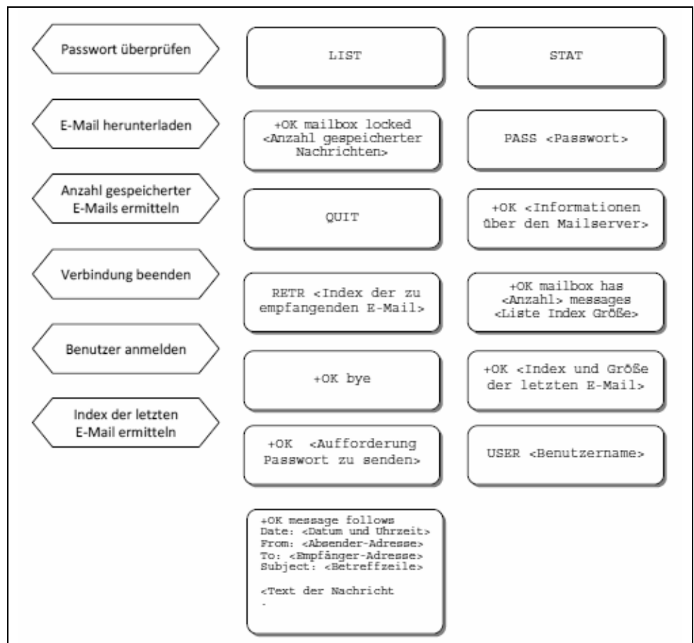
Abbildung 6: Ungeordnete Nachrichten und Schritte der Kommunikation zum Abrufen neuer E-Mails.
